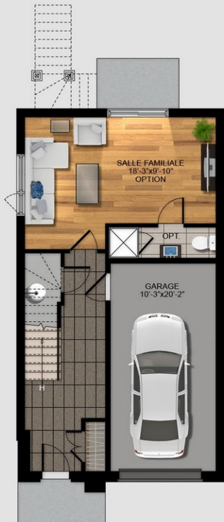
REZ-DE-JARDIN 195 pi 2 (vestibule et passage)
